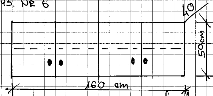
SZAFKA WISZĄCA - szt. 1
