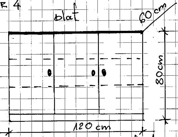
SZAFKA BIUROWA - szt. 1 dwiczki zamknięte na klucz
